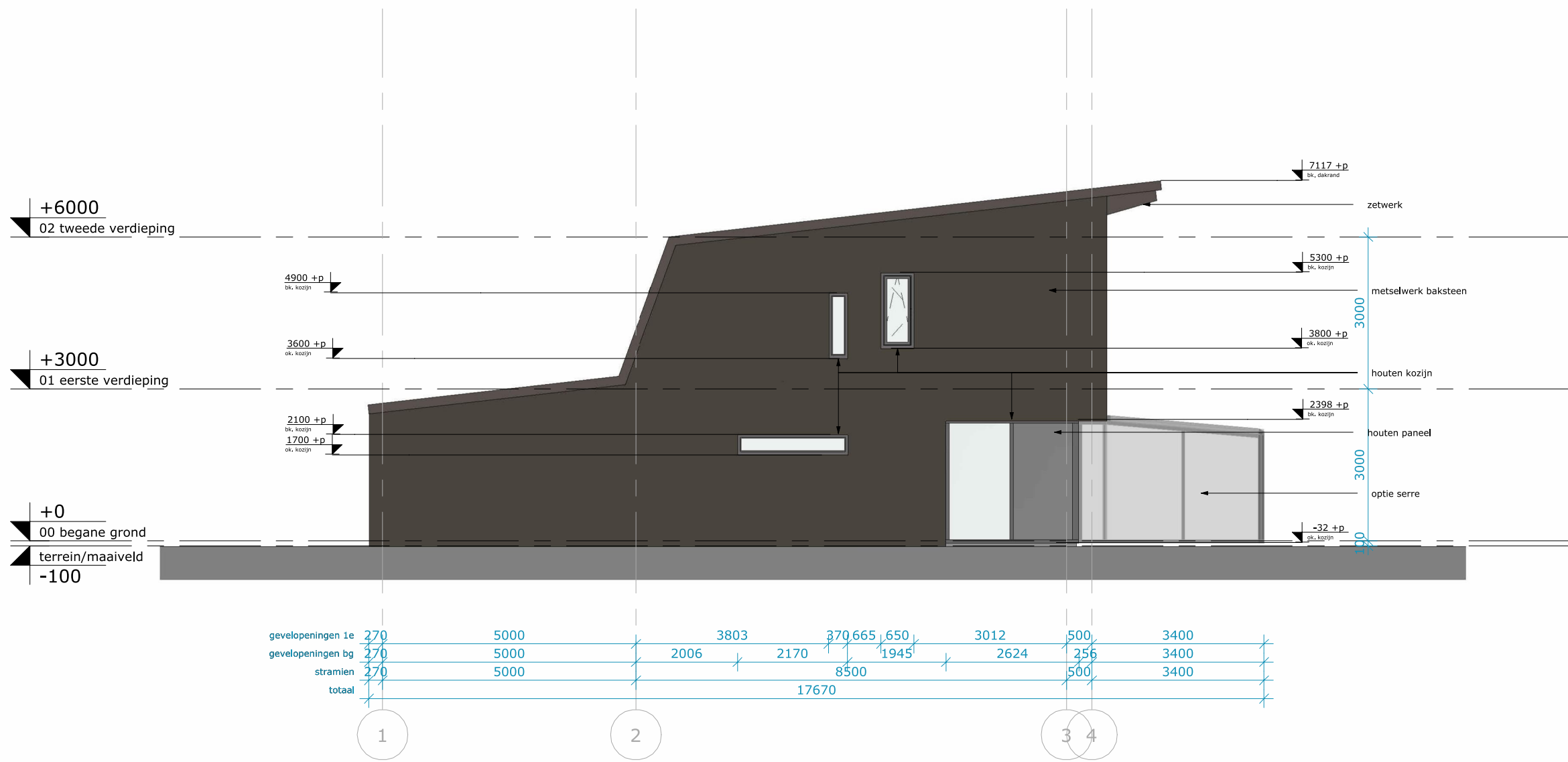
Rechterzijgevel
