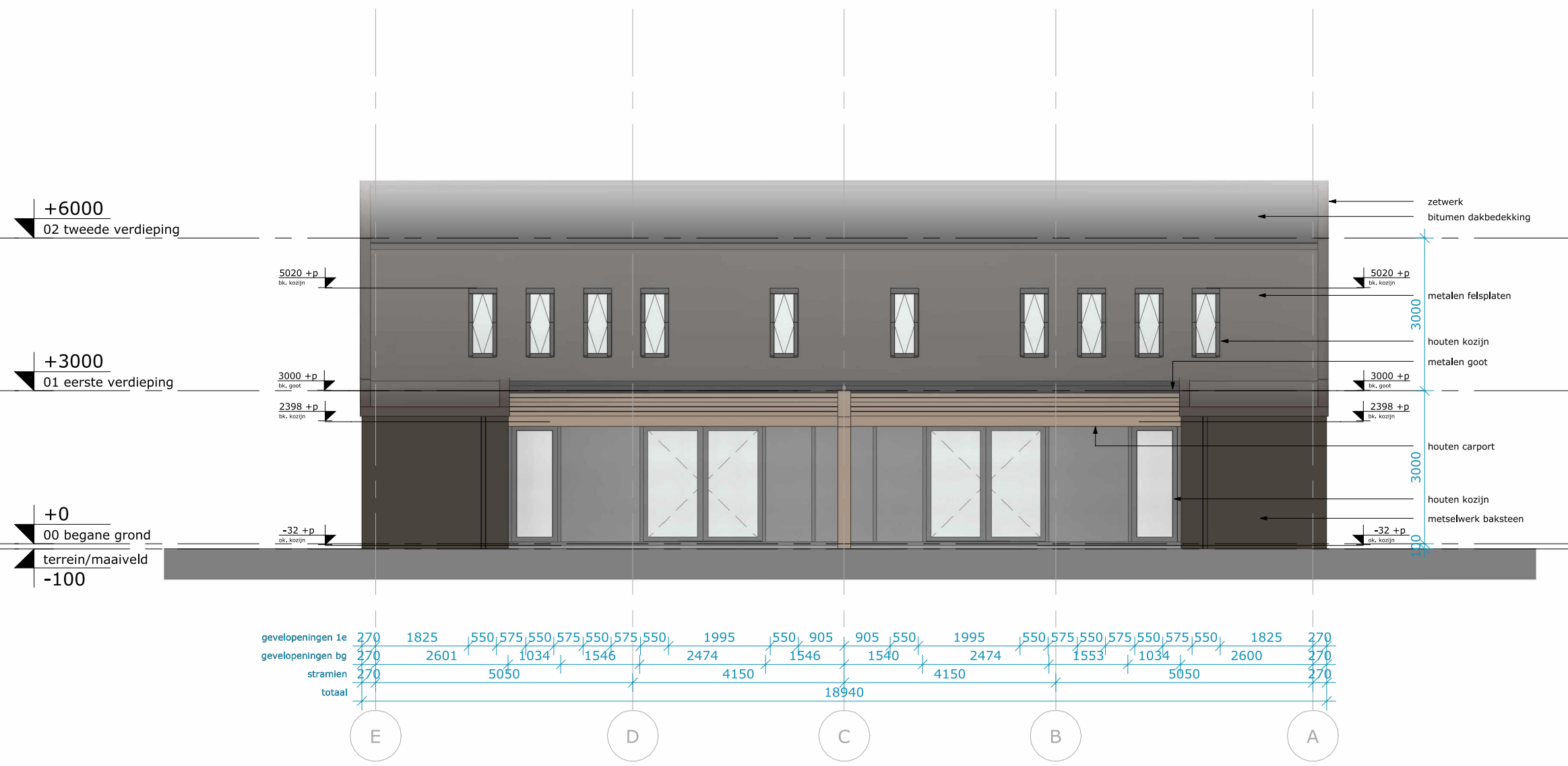
Voorgevel
