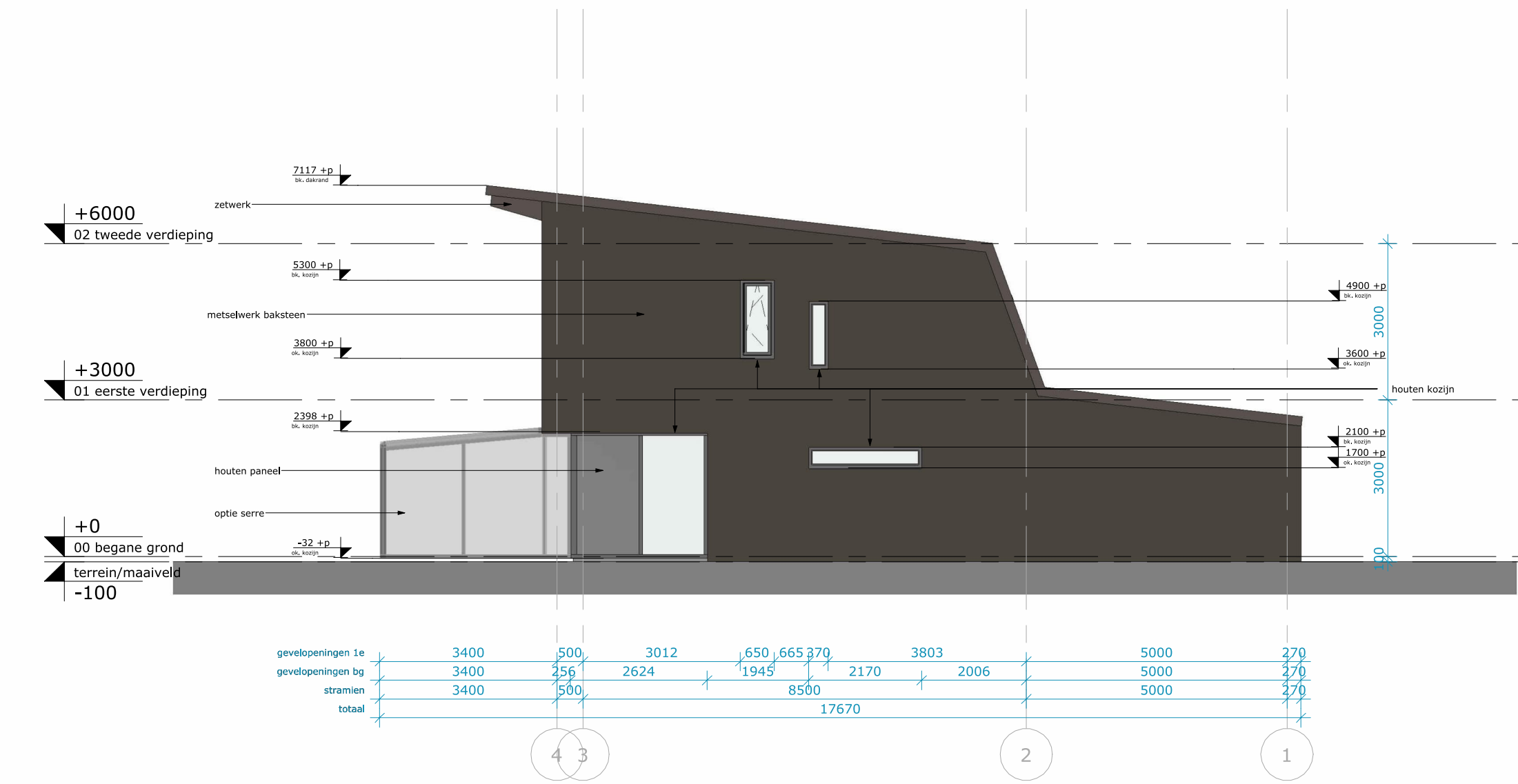
Linkerzijgevel
