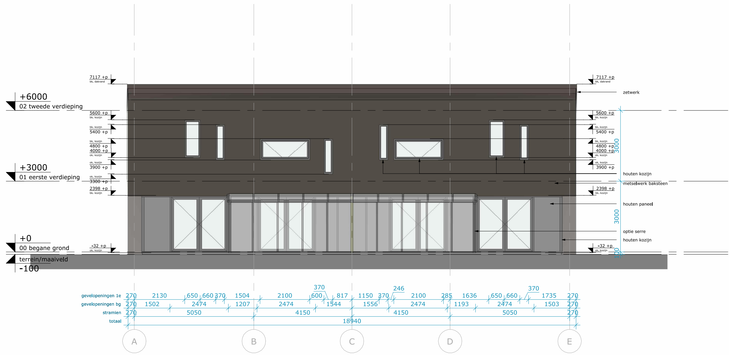
Achtergevel
