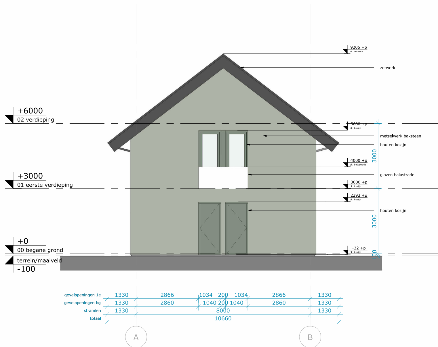
Rechterzijgevel
