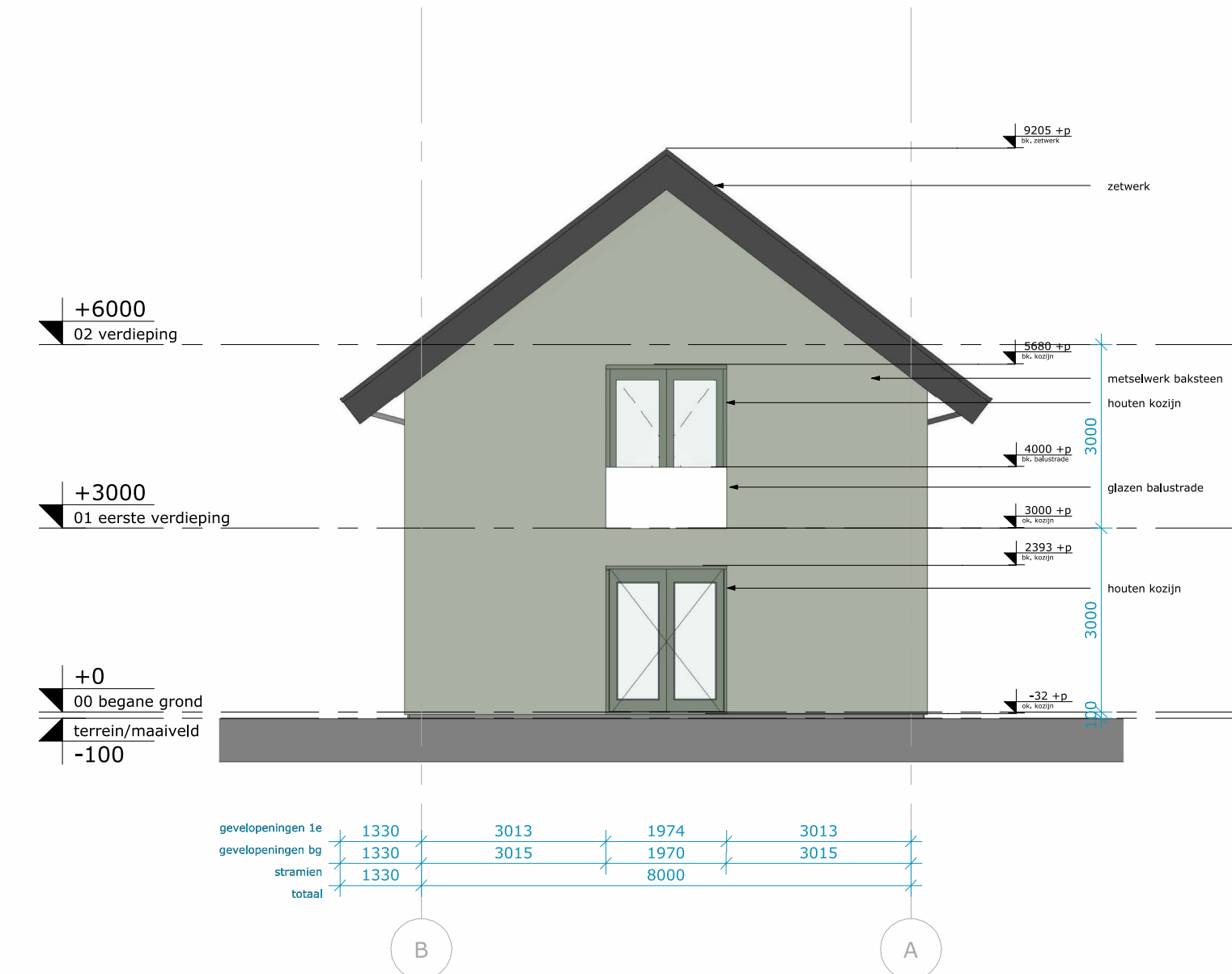
Linkerzijgevel
