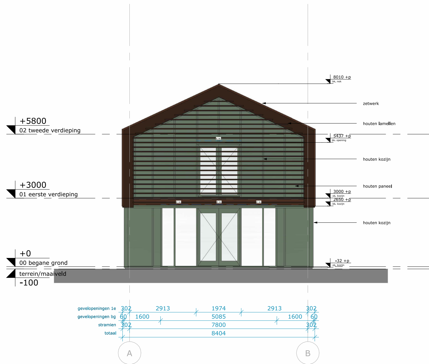
Linkerzijgevel
