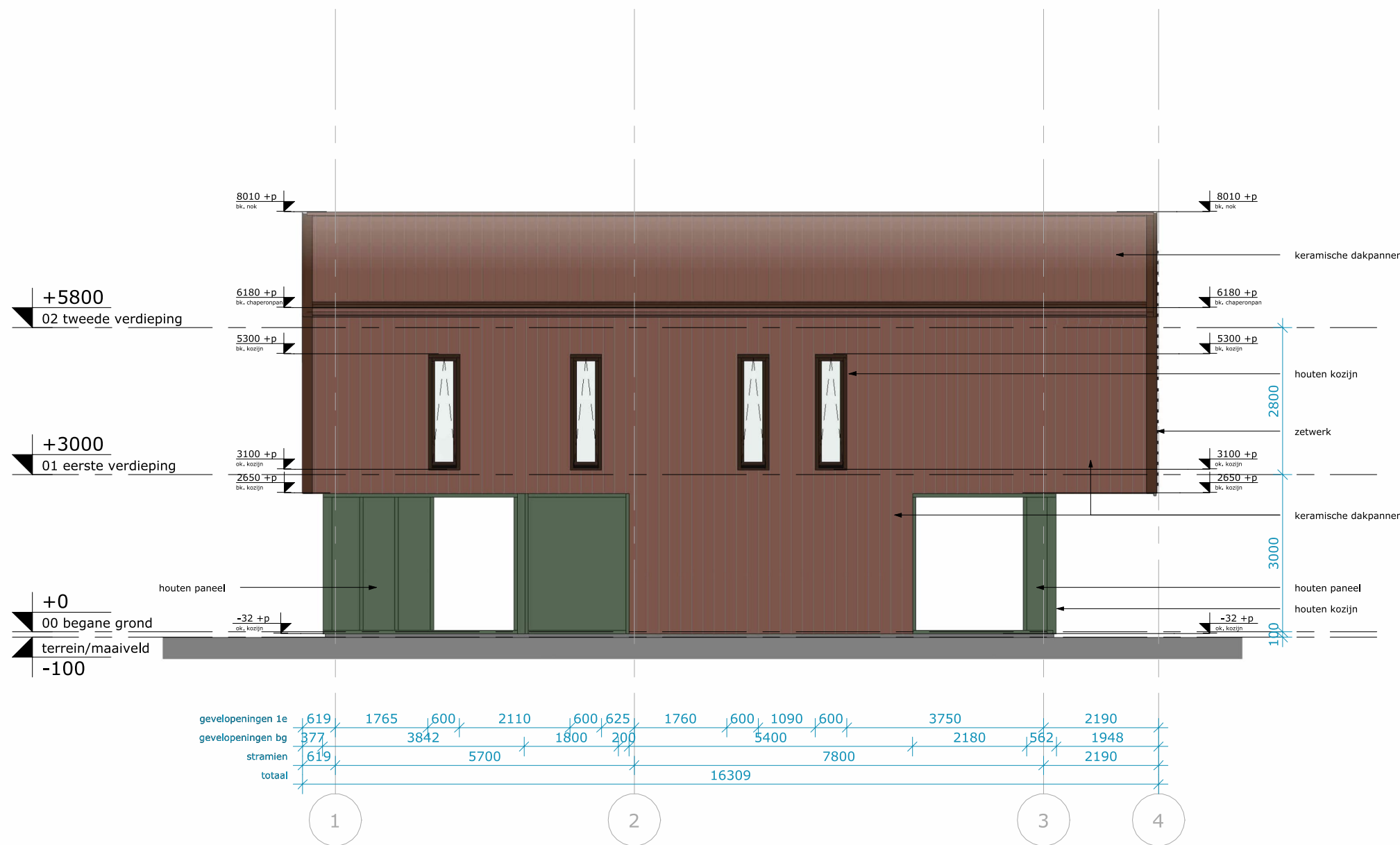
Achtergevel
