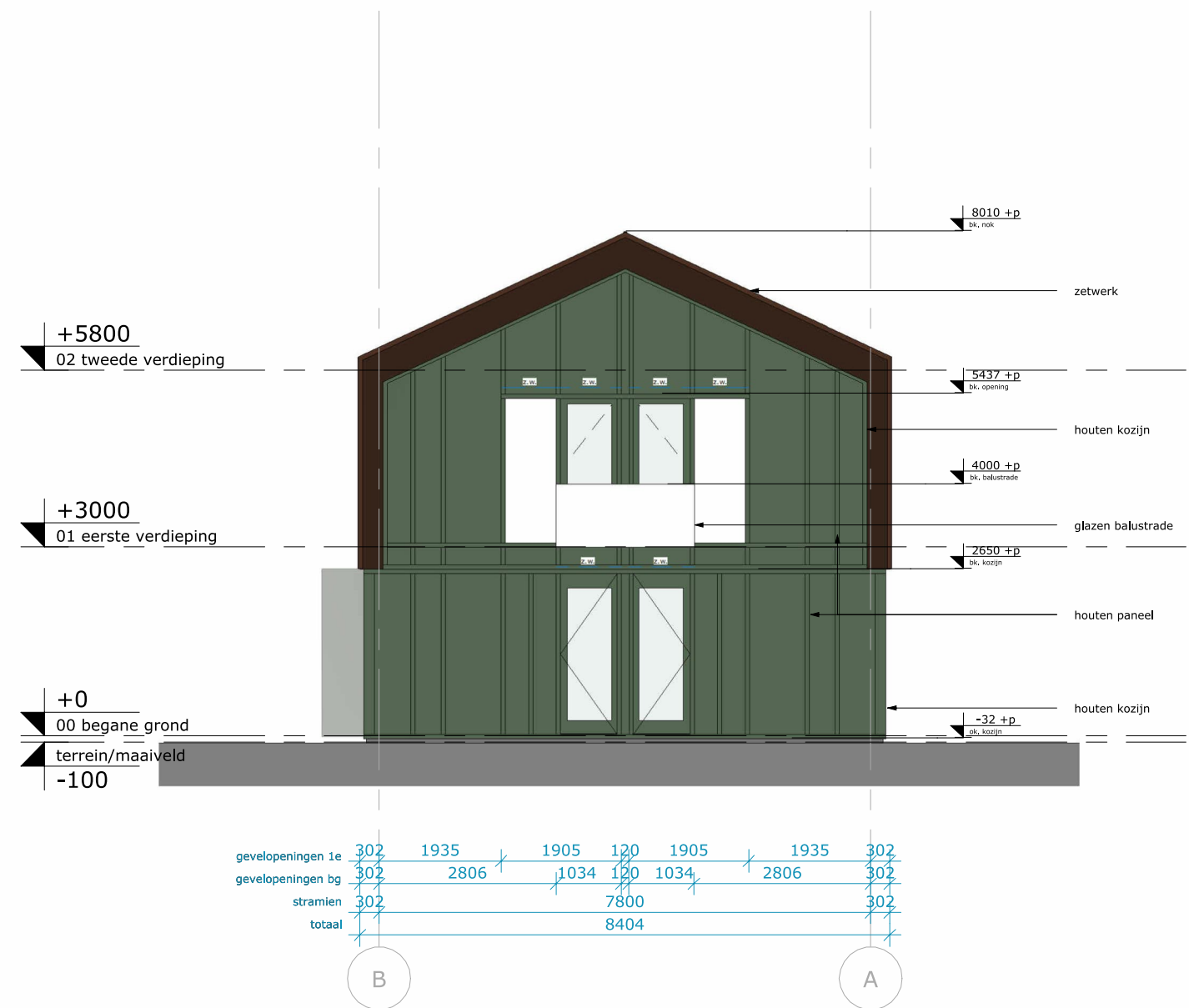
Rechterzijgevel
